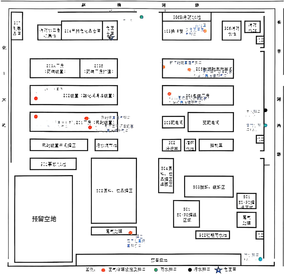
南京威尔生物科技有限公司平面布置图
